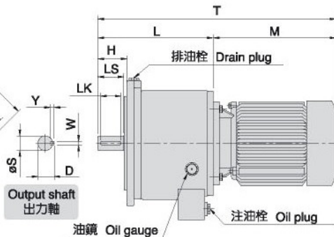
尺寸表 Dimension
